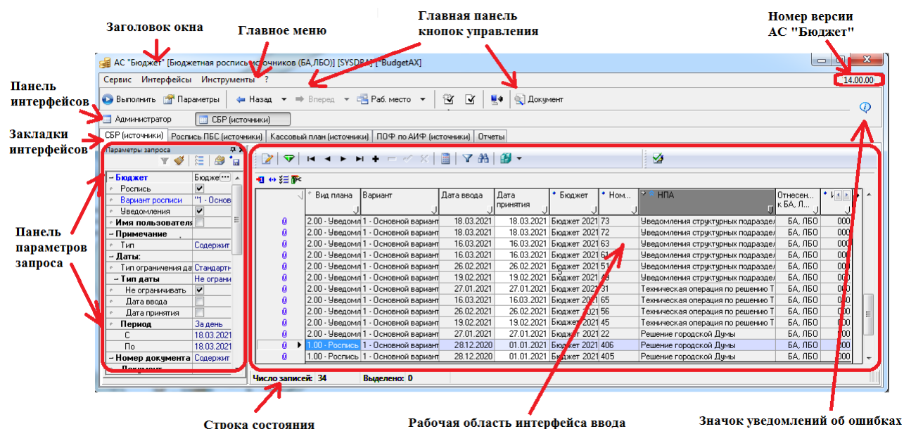
Рис. 2.1 Вид основного окна АС «Бюджет»
