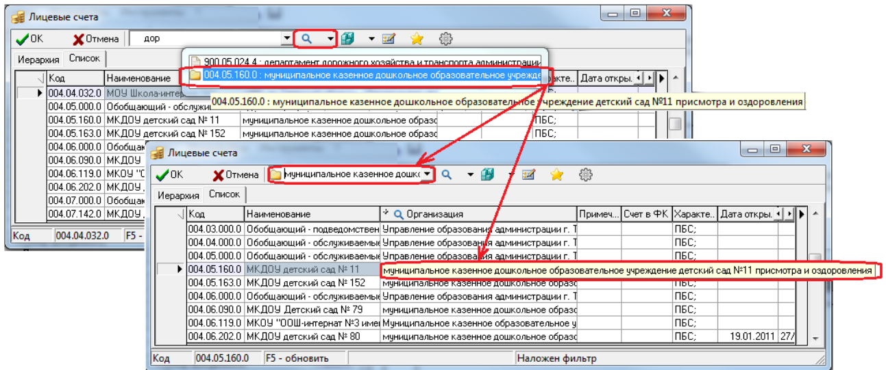
Рис. 4.38 Выполнение поиска значения классификатора «Лицевые счета» путем выбора нужного значения из выпадающего списка автозавершения поля «Организация»
